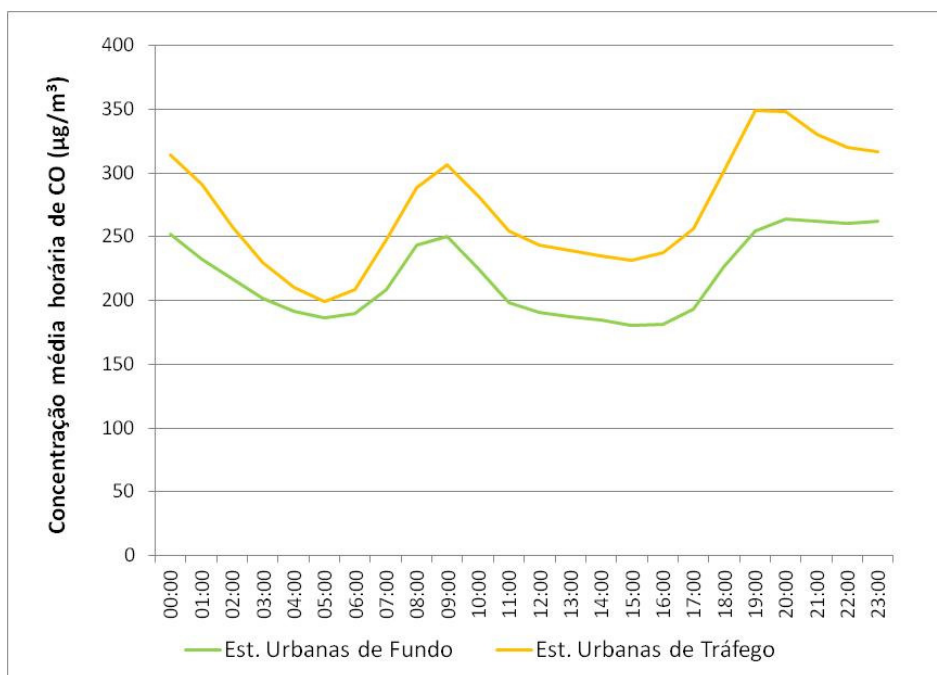
Figura 21. Ciclo diário das concentrações de CO nas estações urbanas de fundo e estações de tráfego da RMQA LVT
