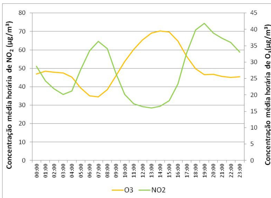
Figura 30. Ciclo diário das concentrações de NO 2 e O 3 na estação dos Olivais
