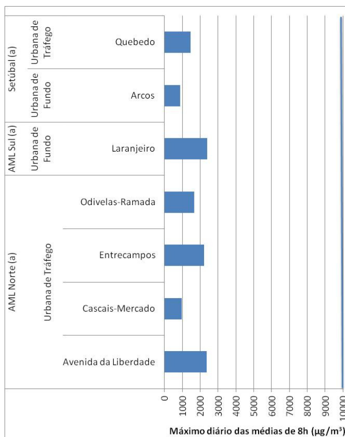
Figura 22. Avaliação da conformidade legal do poluente CO em 2015, para a proteção da saúde humana
