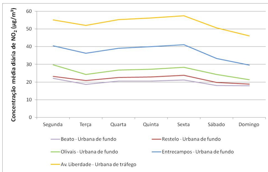
Figura 5. Ciclo semanal das concentrações de NO 2 nas estações da AML Norte
