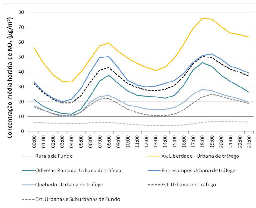
Figura 4. Ciclo diário das concentrações de \text{NO}_2 nas estações da RLVT
