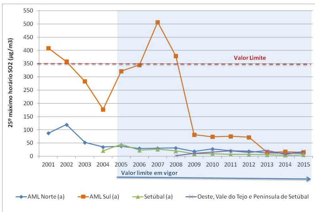
Figura 26. Evolução do 25º máximo horário de SO 2 nas zonas da RLVT (valor máximo das estações de cada zona)
