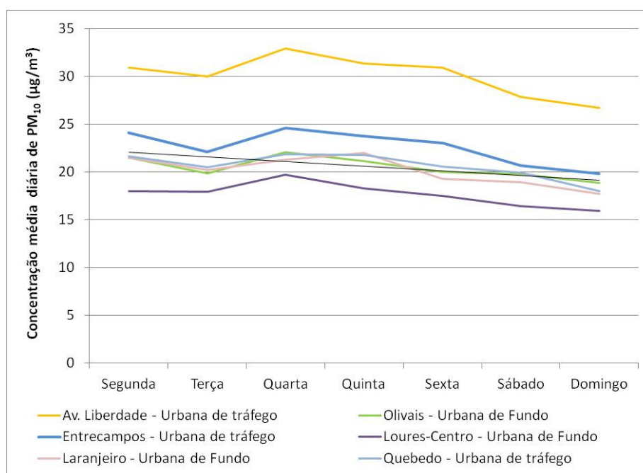
Figura 13. Ciclo semanal das concentrações de PM 10 em estações das aglomerações da RLVT
